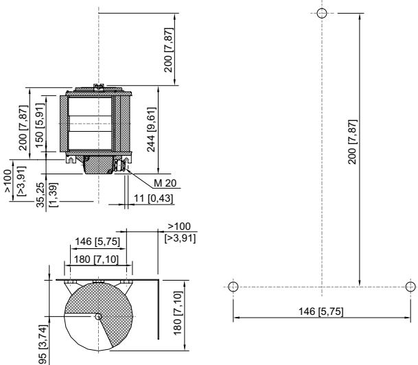
TEF 2850 Sektorlaterne
