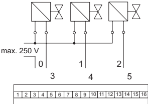
Anschlussplan 9477/12-08-12
