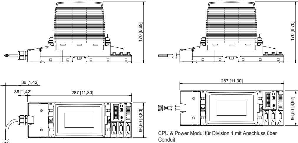
CPU & Power Modul für Zone1 mit Anschluss über Kabelschwanz
