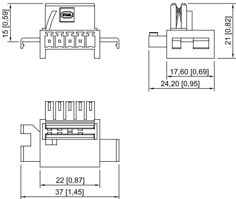
Reihe 9194
