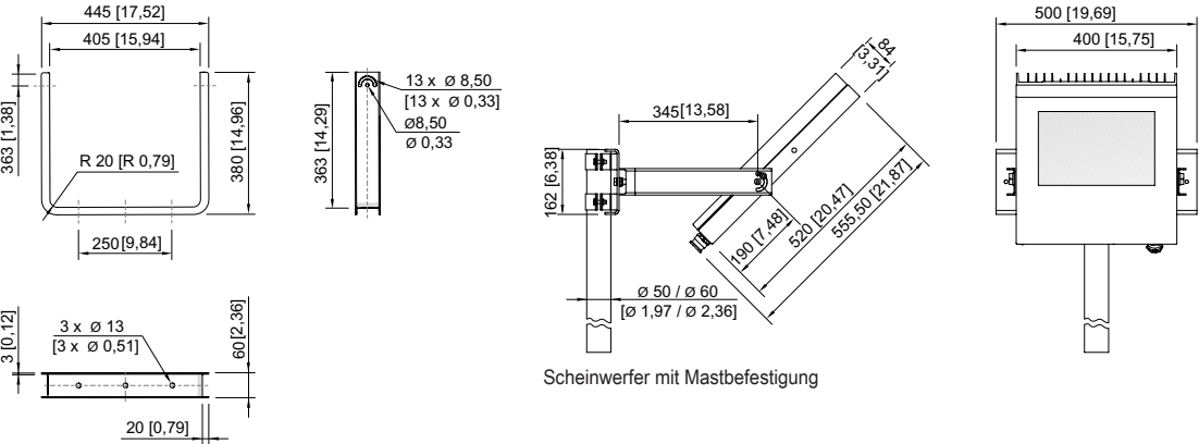
Montagebügel
