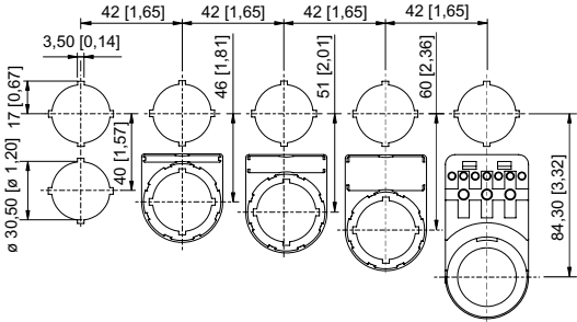
Einbaustermaß mit / ohne Zusatz- Bezeichnungsschild
