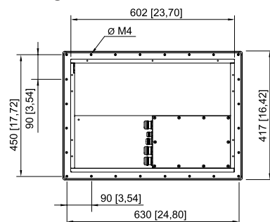
Schalttafel-Einbaumodul Rückansicht
