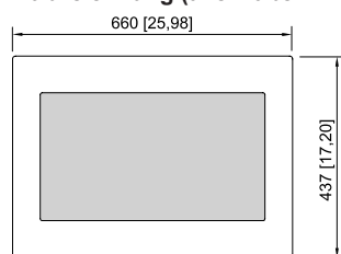
Schalttafel-Einbau Ansicht vorn
