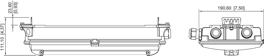
mit Befestigungsbügel
