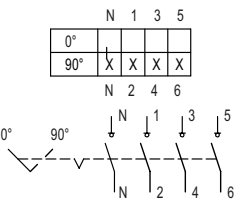
Schaltabwicklung 8544/1-4 und 8549/1-4
