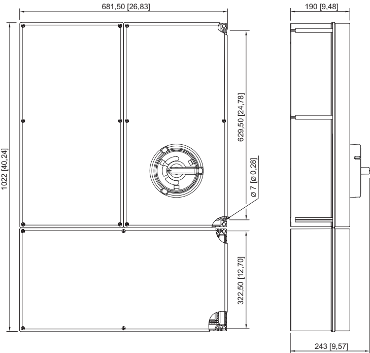
Maßzeichnung (alle Maße in mm [Zoll]) – Änderungen vorbehalten
