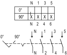
Schaltabwicklung 8544/1-4 und 8549/1-4
