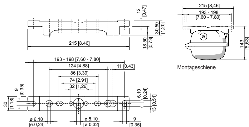
Montageschiene
