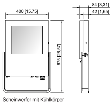
Scheinwerfer mit Kühlkörper
