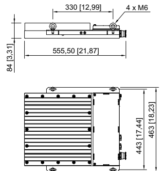
Scheinwerfer mit Kühlkörper, mit Ringösen
