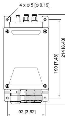
Inneneinbau-Set Typ 8622/68 für Ex p Controller
