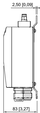
Inneneinbau-Set Typ 8622/68 für Ex p Controller
