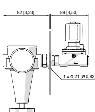
Ex p Spülventil mit Druckregler R 1/2" Typ 8622/21
