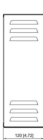
IP66 Wirbelstrom-Luftkühler-Haube Typ 8622/64
