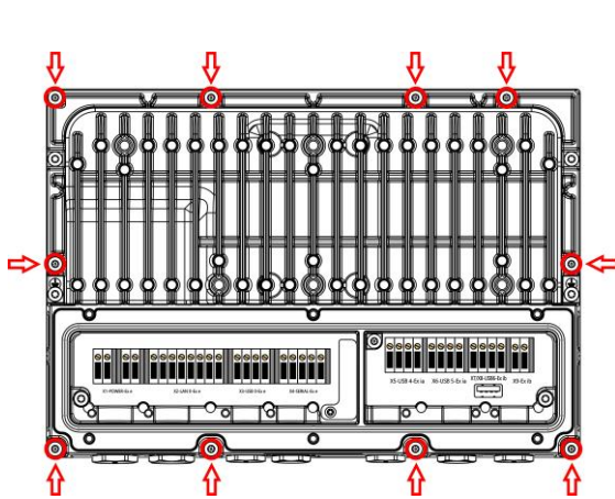
E-Box 标准后视图
