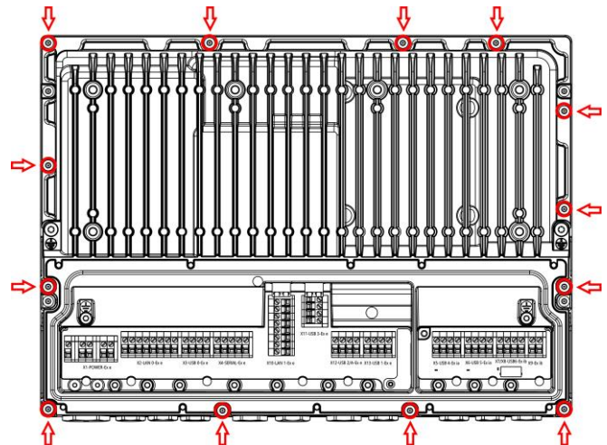
E-Box PRO 后视图
